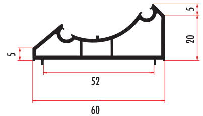
YARA601 60 MM KÖŞE DÖNÜŞ ADAPTÖRÜ CORNER ADAPTOR FOR 60 MM SERIE YARA602 (RENKLİ/COLORED)
