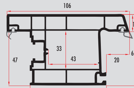
PEG62461 62 MM - 3 ODACIKLI DIŞA AÇILIR KAPI KANAT / OUTWARD OPENING DOOR SASH PROFILE PEG62462 (RENKLİ/COLORED)
