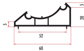
YARA601 60 MM KÖŞE DÖNÜŞ ADAPTÖRÜ CORNER ADAPTOR FOR 60 MM SERİE YARA602 (RENKLİ/COLORED)
