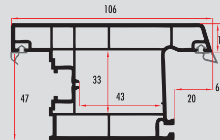
PEG62461 62 MM - 3 ODACIKLI DIŞA AÇILIR KAPI KANAT / OUTWARD OPENING DOOR SASH PROFILE PEG62462 (RENKLİ/COLORED)
